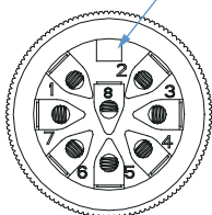
Positionierungsschlitz
