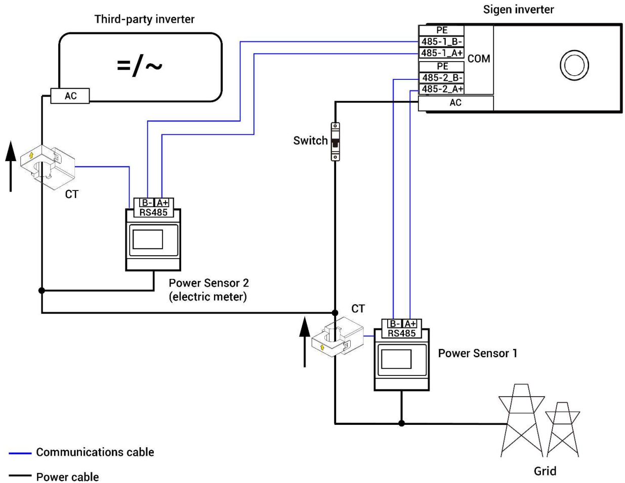
Figure 2-3 Diagramm der Verdrahtungsverbindungen von Wechselrichtern von Drittanbietern
