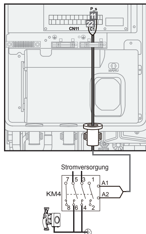
Solarenergiepumpe P_s:
