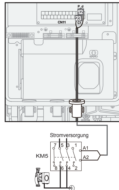
WW-Rohrpumpe P_d:
