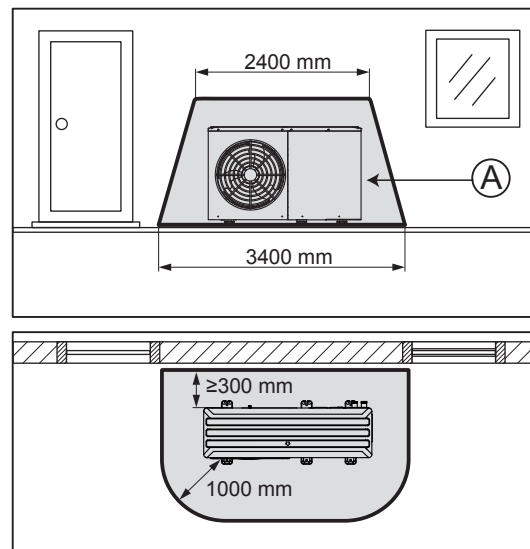
Aufstellen des Außengeräts vor einer Außenwand
